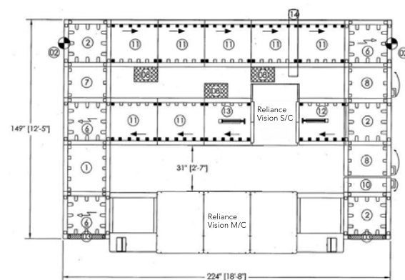
Layout típico/configuração
